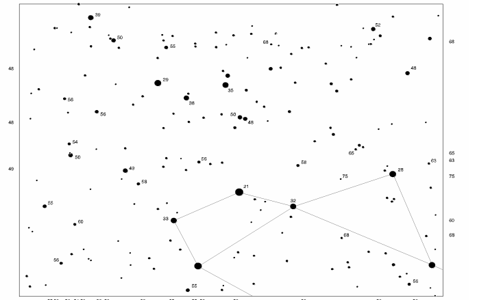
Grenzgrößenkarte 4 Sagittarius
