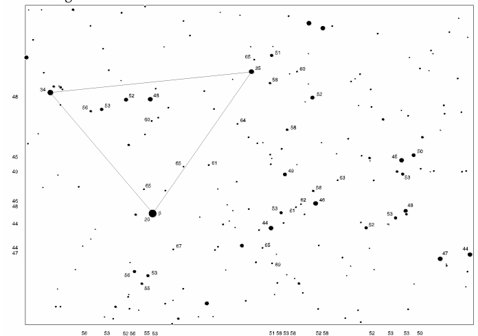
Grenzgrößenkarte 6 Cetus
