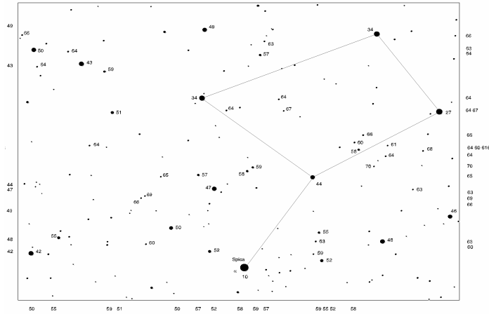
Grenzgrößenkarte 2 Virgo
