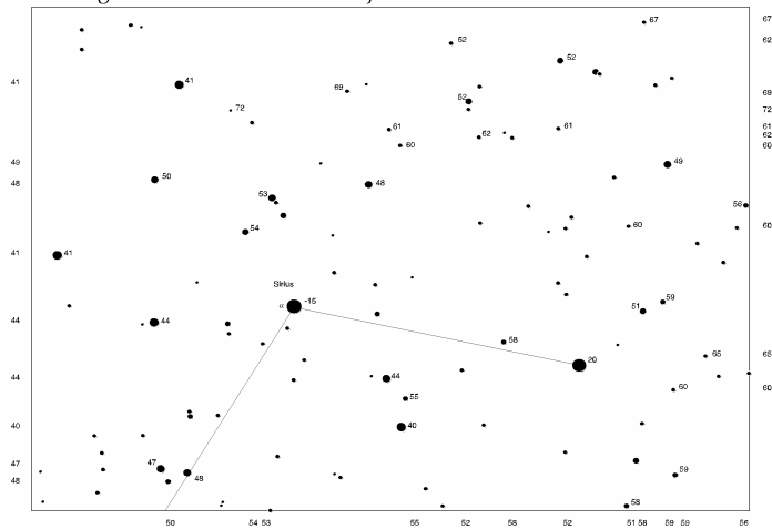
Grenzgrößenkarte 8 Canis Major
